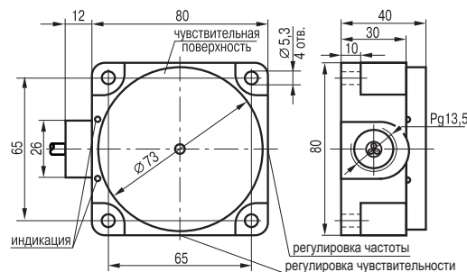
Габаритный чертёж
